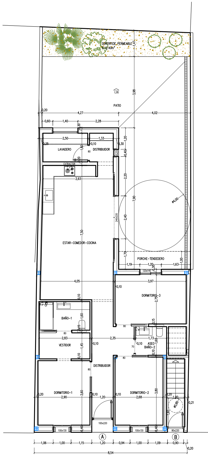
PLANTA BAJA -COTAS-
