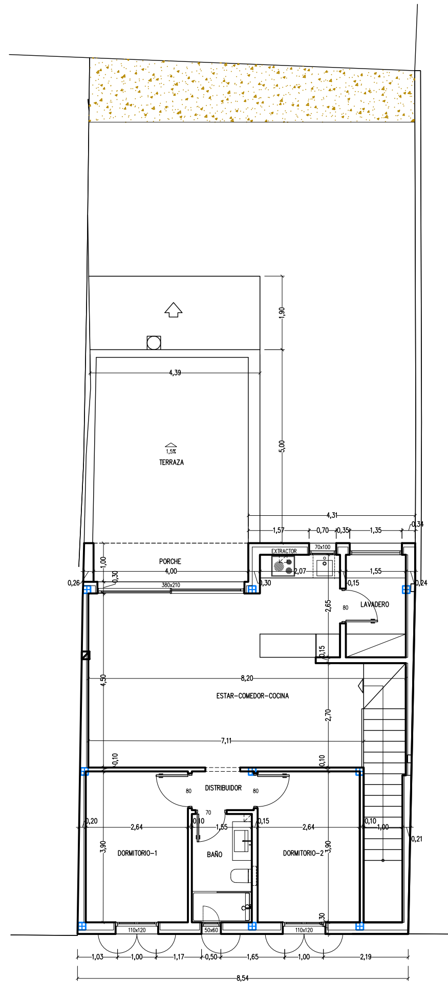
PLANTA PISO 1 -COTAS-
